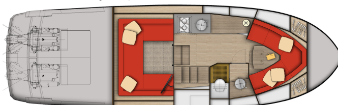
Nenhum camarote: versão "LOUNGE"
