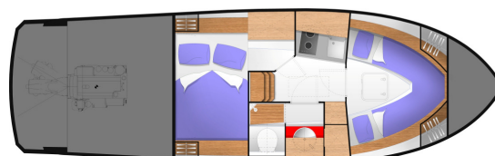
Camarote a meia-nau fechado e camarote na proa fechado, com 2 camas de solteiro
